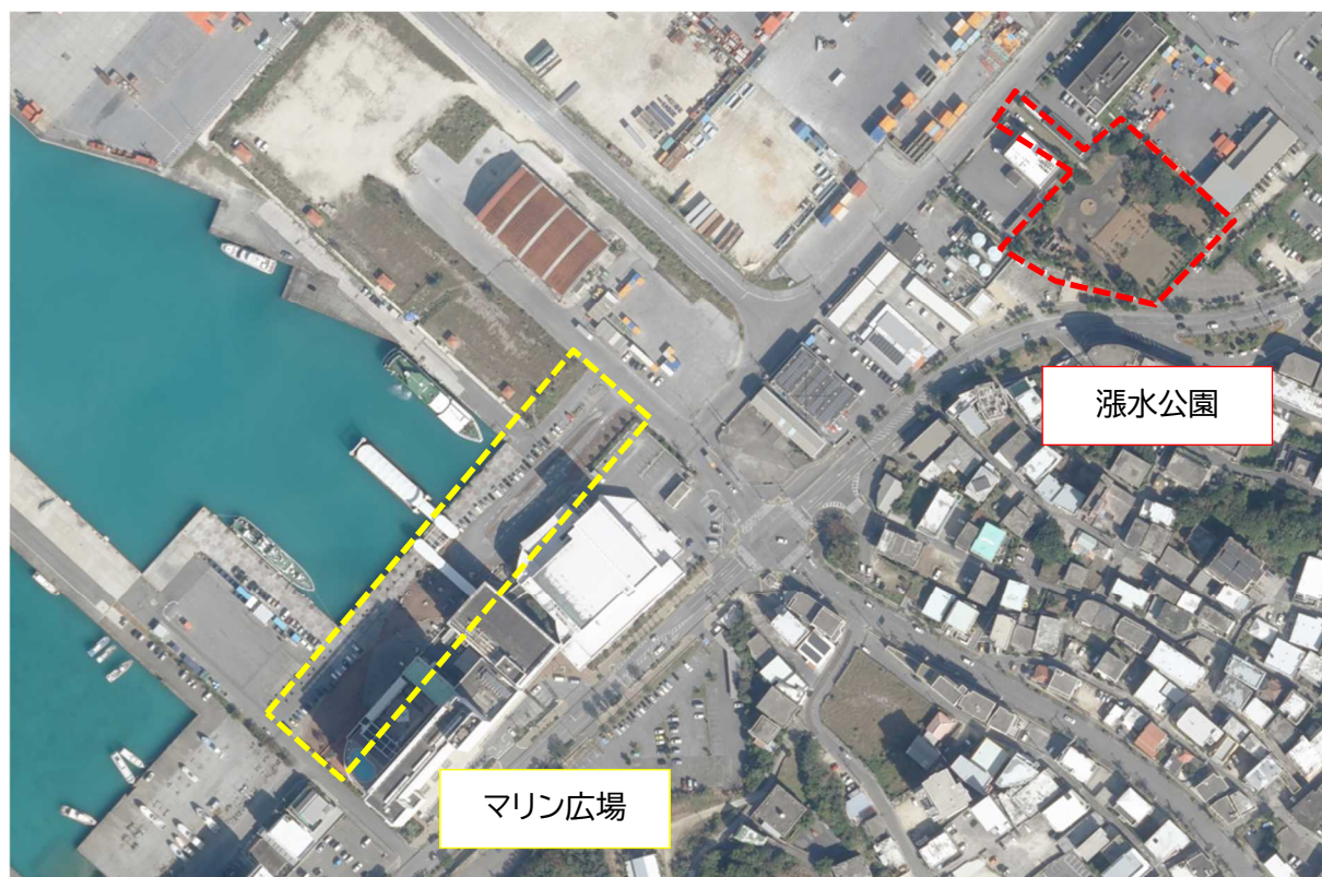
作業箇所図（臨港道路伊良部線）
