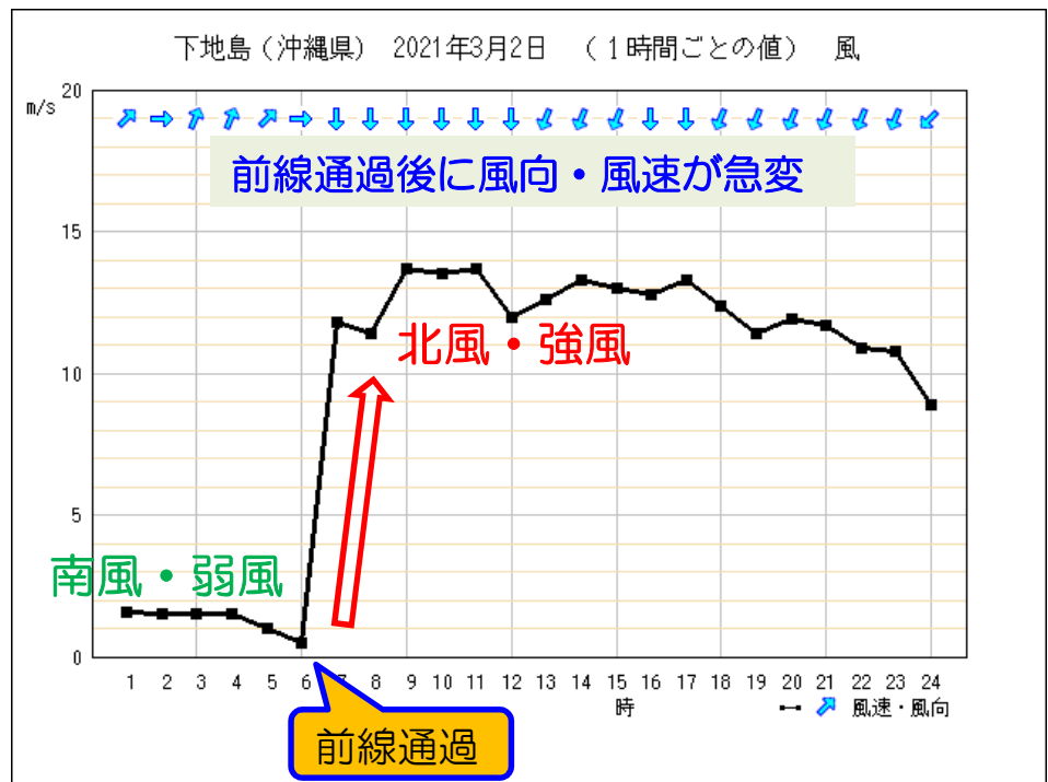
図：2021年3月2日3時の天気図（左上）、9時の天気図（左下）、下地島の風向・風速（右）
