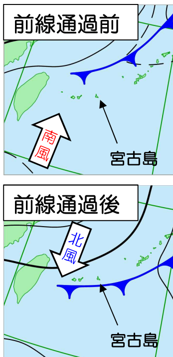
図：2021年3月2日3時の天気図（左上）、9時の天気図（左下）、下地島の風向・風速（右）
