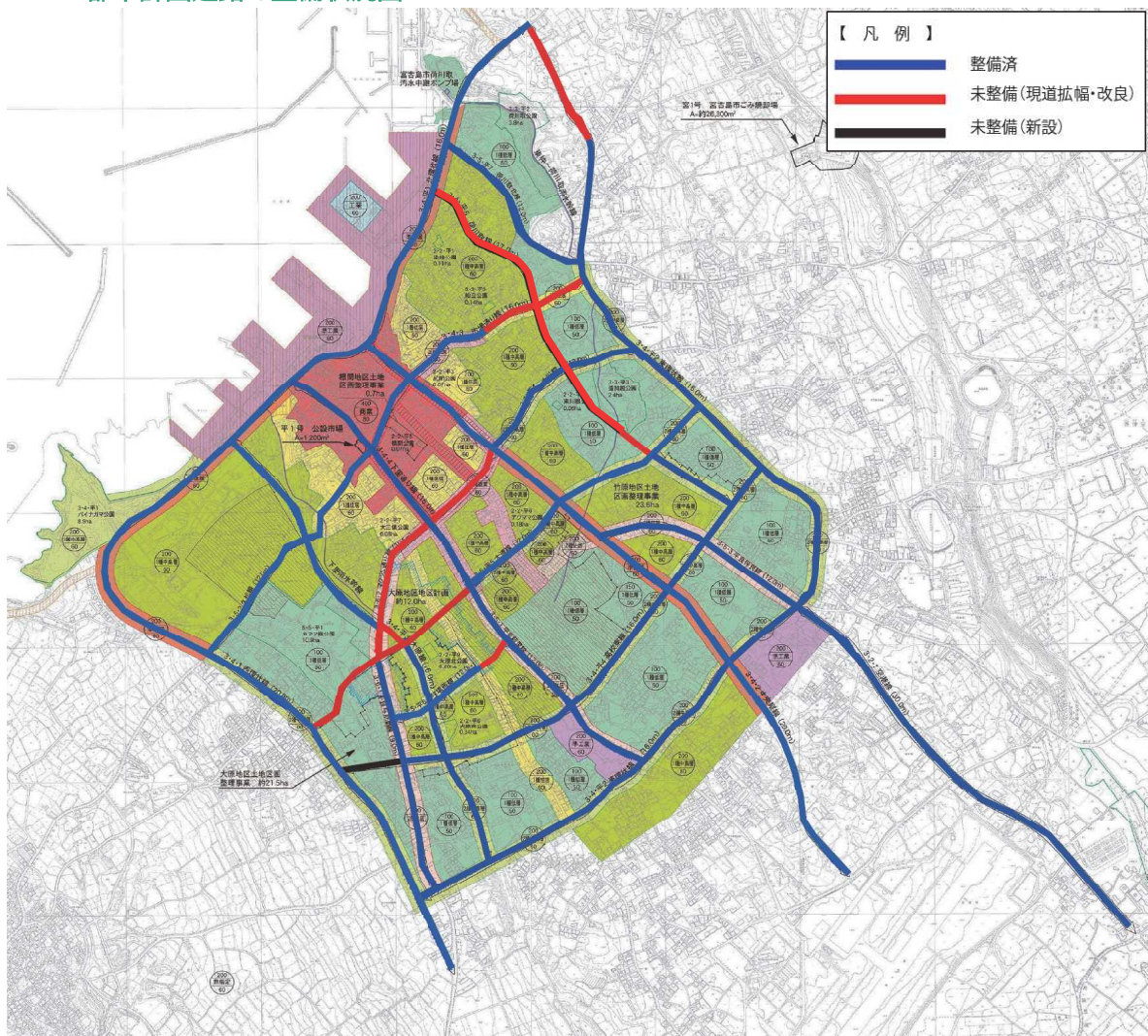
■都市計画道路の整備状況図
